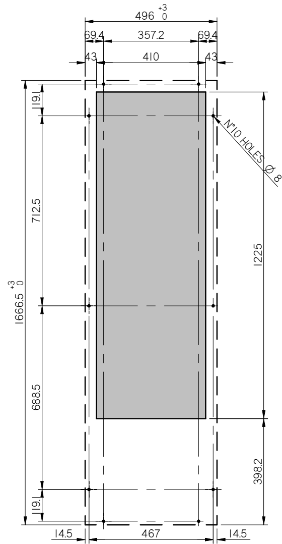
MONTAGGIO ESTERNO EXTERNAL MOUNTING
