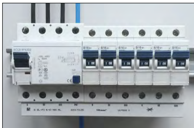
Verdrahtung mit Phasenschiene connection with busbars connexion avec peigne
